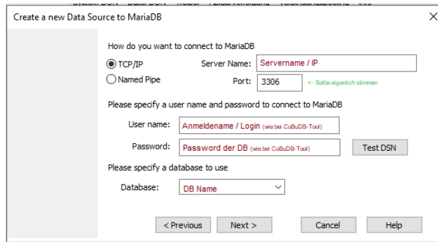
Abbildung 5: ODBC Ansicht 2
