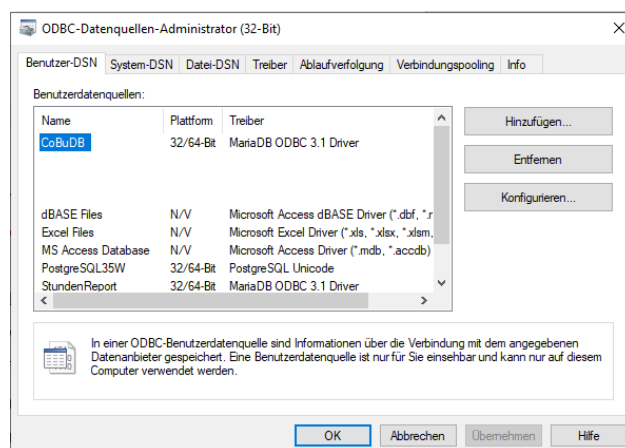
Abbildung 3: ODBC Ansicht
