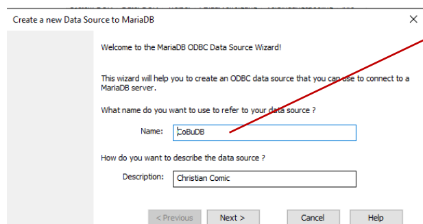
Abbildung 4: ODBC Ansicht 1
